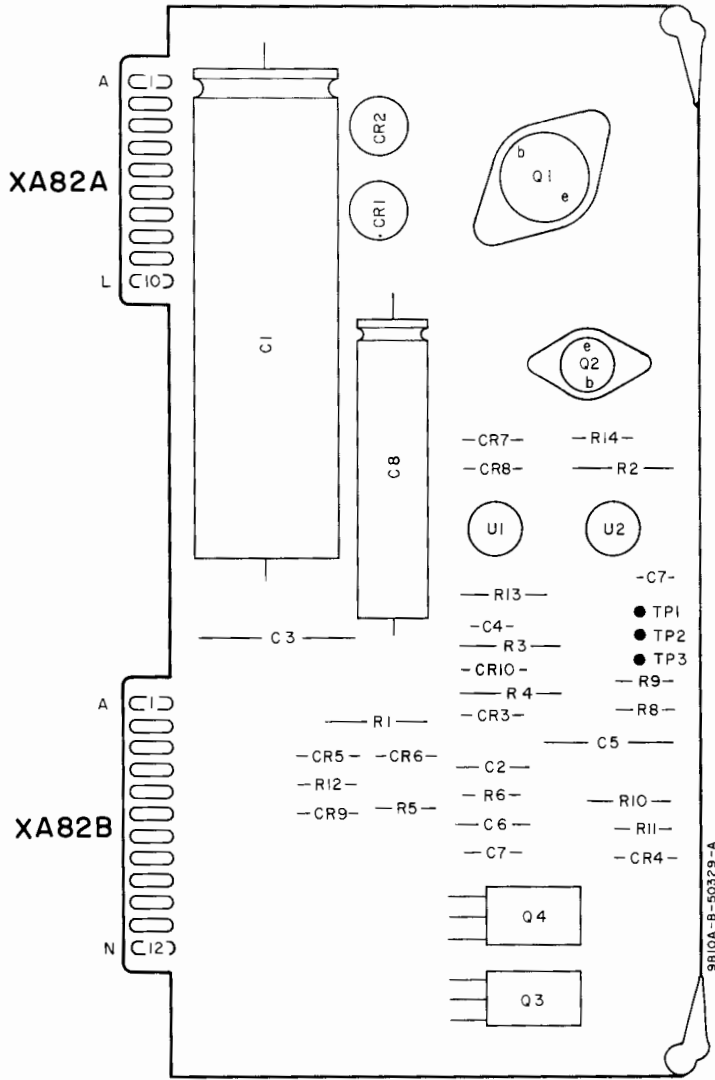
A82 hp Part No 09810-66582 REV A
