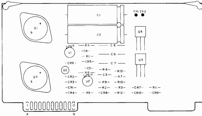
A83 hp Part No 09810-66583 REV A
